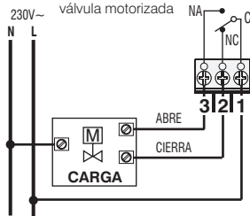
Conexión a una válvula motorizada
