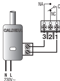
Conexión a una caldera
